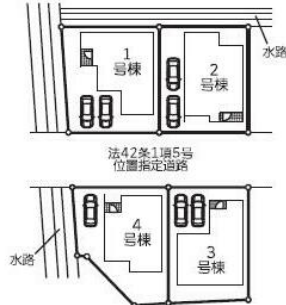
間取図（平面図）
