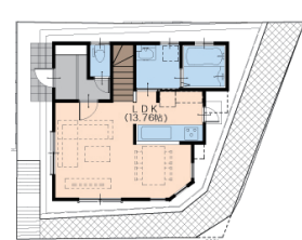
1階 平面図
